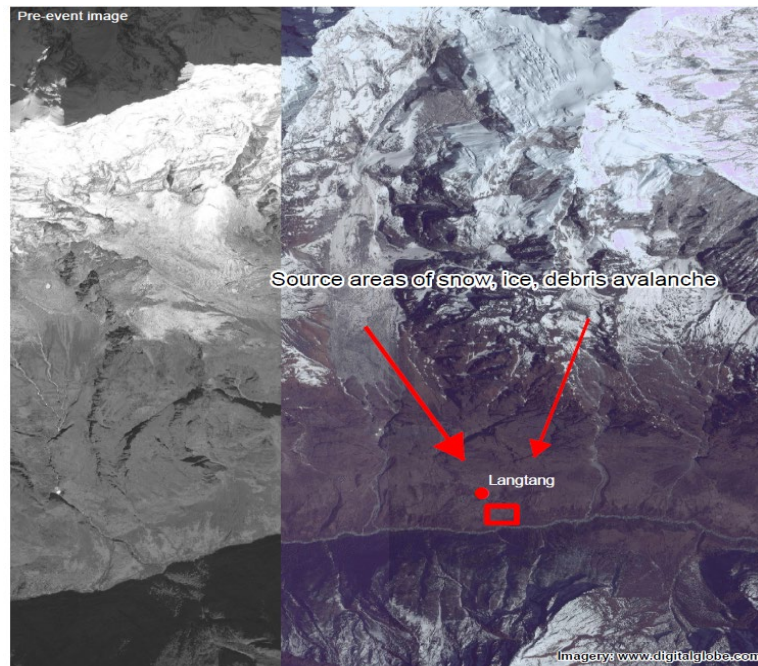
圖 10：掩埋 Langtang Village 雪、冰、土石可能來源
