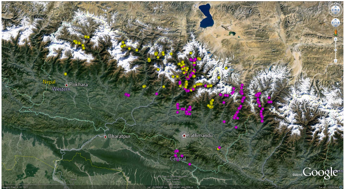
圖 9：尼泊爾地震造成之山崩位置分布
