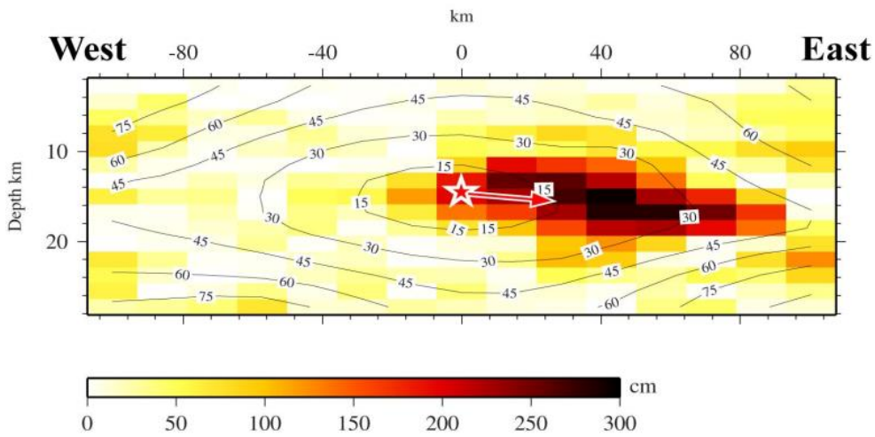
圖 3：本次地震斷層面錯動模擬模型（資料來源：台灣地震科學中心）
