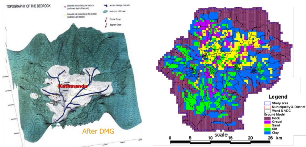
圖 4：(a)加德滿都谷地地形 (b)加德滿都谷地沖積層之土壤性質分布 （資料來源：JICA/MoHA）
