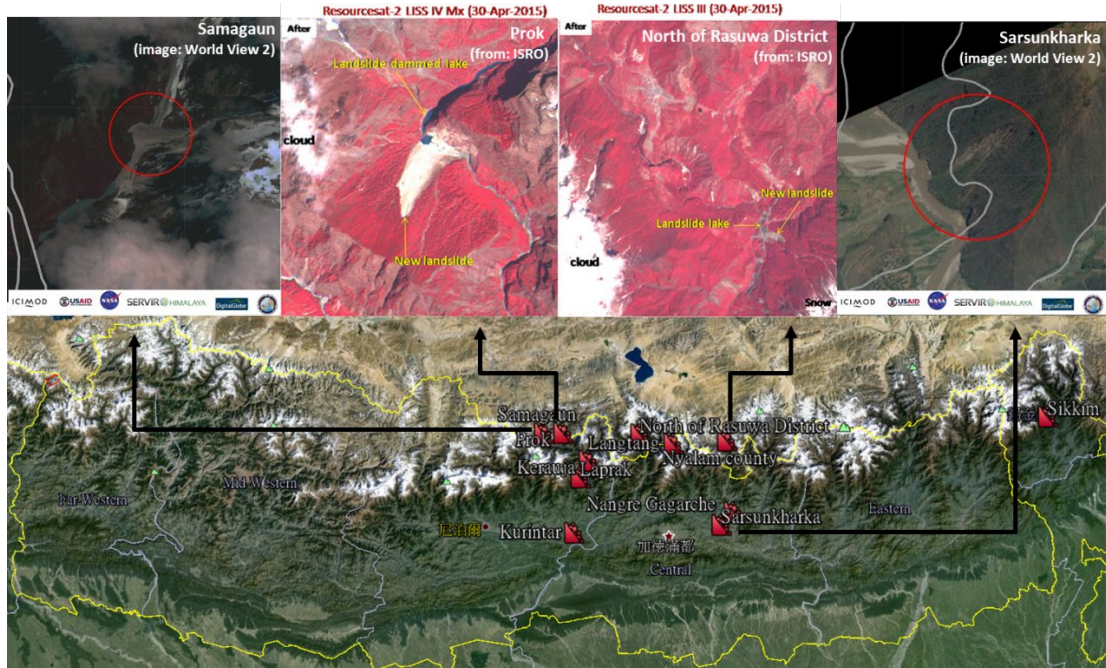
圖 13：部分山崩阻斷河道，可能形成堰塞湖位置
