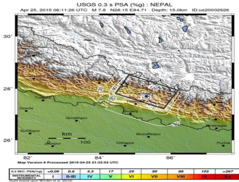
圖 7：本次地震 0.3 秒譜加速度分布圖（資料來源：USGS）
