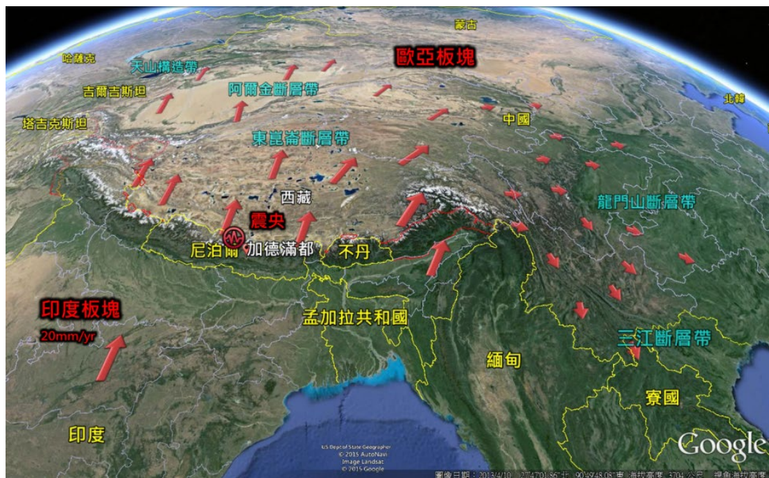
圖 2：尼泊爾鄰近之板塊構造分布圖（資料來源：陳文山教授）
