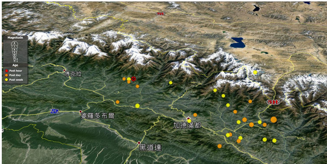
圖 1：尼泊爾地震震央位置（資料來源：USGS）
