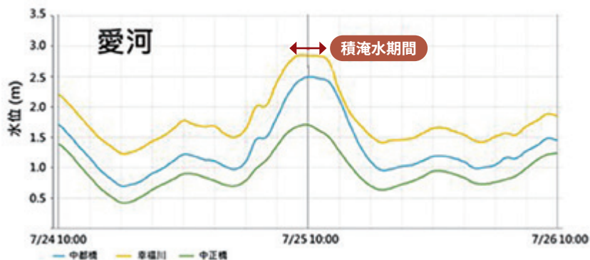
愛河水位觀測站（中都橋、幸福川、中正橋）之觀測紀錄（資料來源：災防科技中心）
