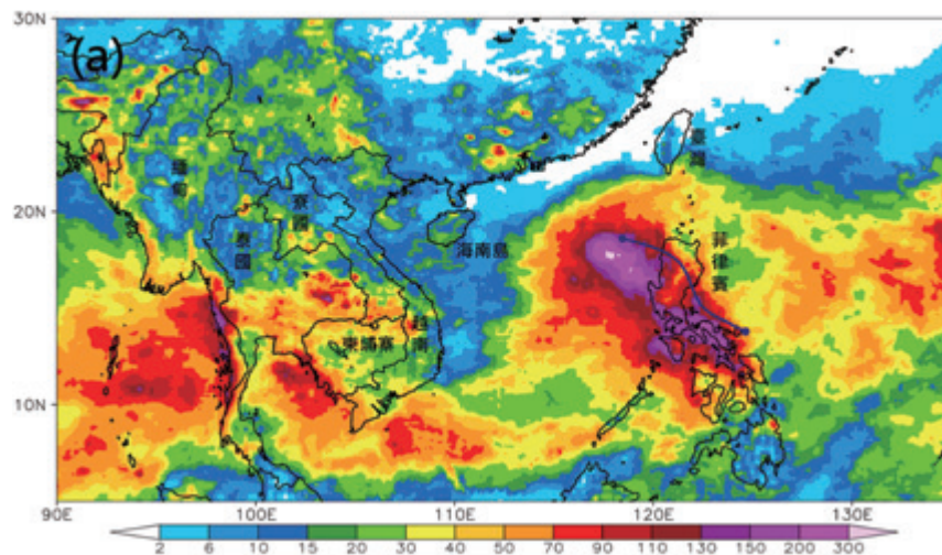
A 9月1日至9月3日累積雨量
