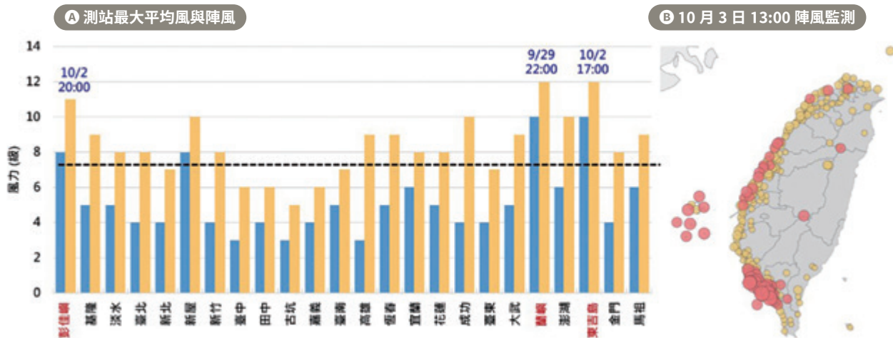
山陀兒颱風影響期間， A 中央氣象署氣象站最大風速及 B 颱風中心登陸時（10 月 3 日 13 時）之自動測站陣風監測 （資料來源：中央氣象署，繪製：災防科技中心）
