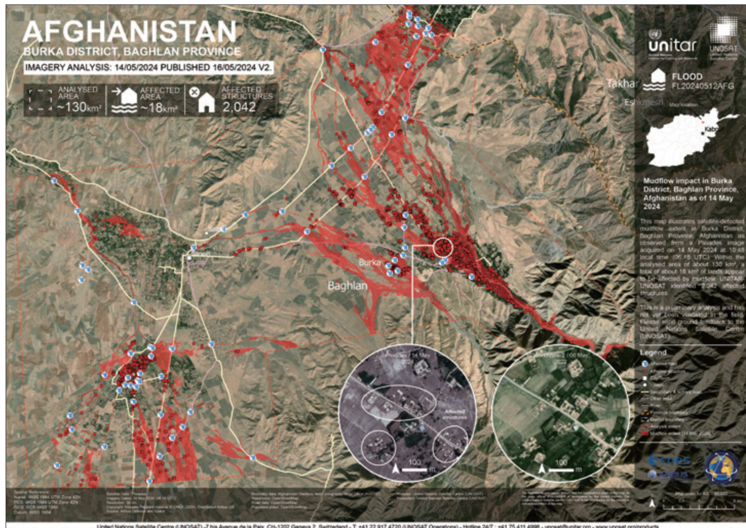
巴格蘭省 Baghlan-e-Jadid 區內的洪水影響區域 (資料來源：UNITAR/UNOSAT)
