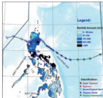
C 銀杏颱風
