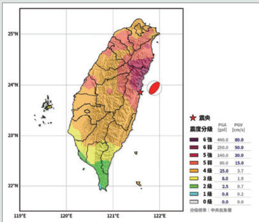
臺灣 0403 主震地表震度圖與震源機制解（資料來源：中央氣象署）
