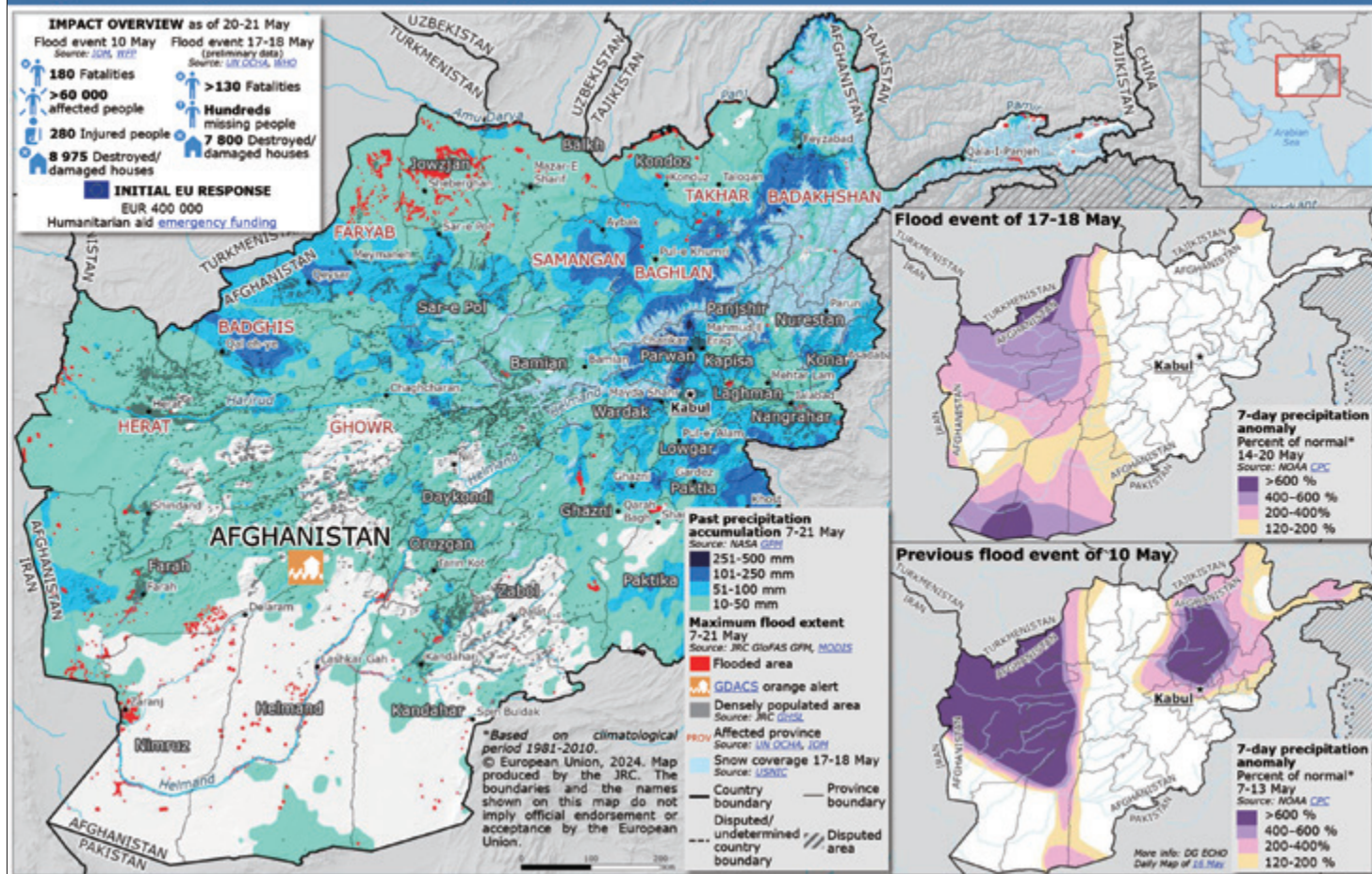
阿富汗 5 月洪水概況與累積雨量距平分布 (資料來源: ERCC)
