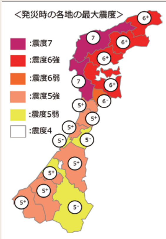
日本能登地震於石川縣最大震度分布圖（資料來源：石川縣政府， 災防科技中心後製）
