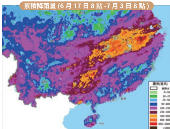
2024 年 6 月 17 日至 7 月 3 日之累積降雨分布 (資料來源：中國氣象局，國家災害防救科技中心重製)
