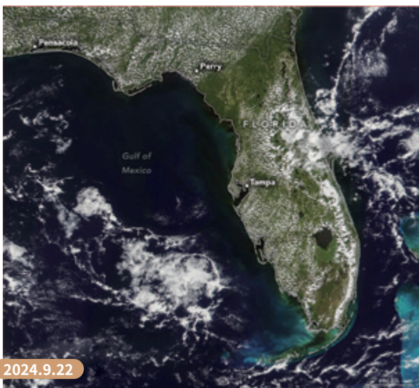
颶風海倫於佛羅里達州墨西哥灣海岸地區之衛星影像分析 (資料來源：NASA)
