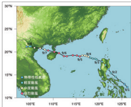
摩羯颱風路徑圖，圖中日期標示點位為每日 00UTC，臺灣時間為 UTC+8。(資料來源：中央氣象署。繪製：國家災害防救科技中心)
