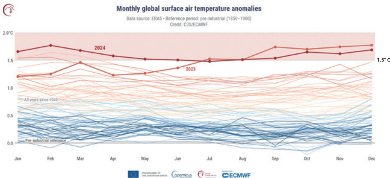
全球地表月均溫距平 (資料來源: ECMWF)
