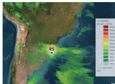
巴西南里約格蘭德州連續降雨事件成因與日累積降雨資料 (資料來源: G1、NASA)
