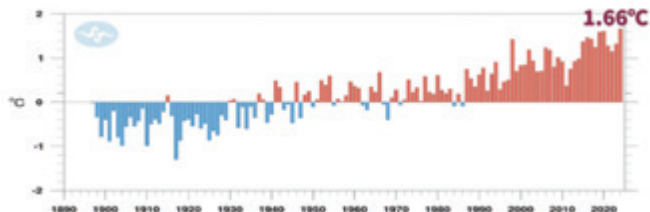
臺灣 1 月至 12 月六個百年測站平均氣溫距平 (資料來源：中央氣象署)
