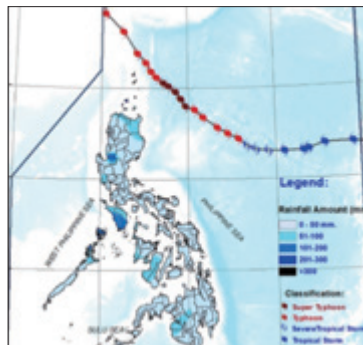
D 桔梗颱風
