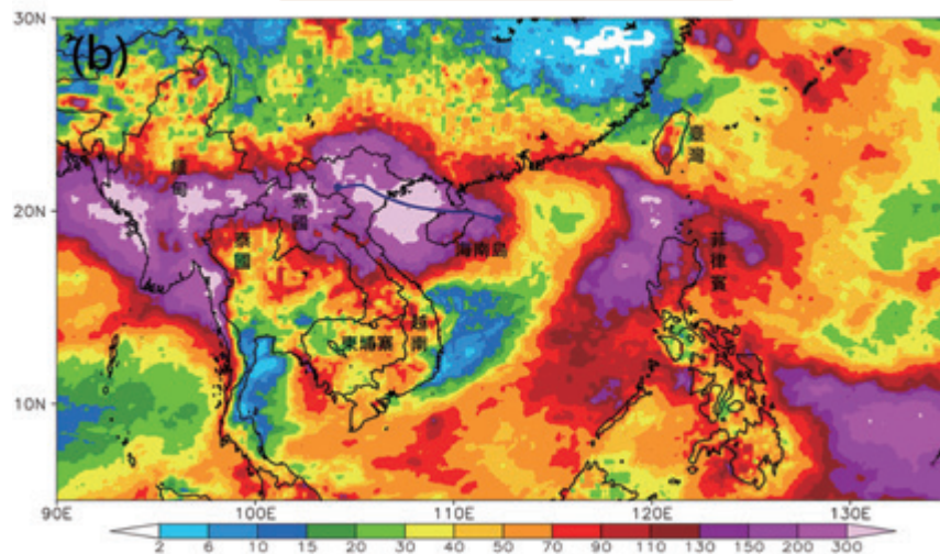
B 9月6日至9月12日累積雨量
