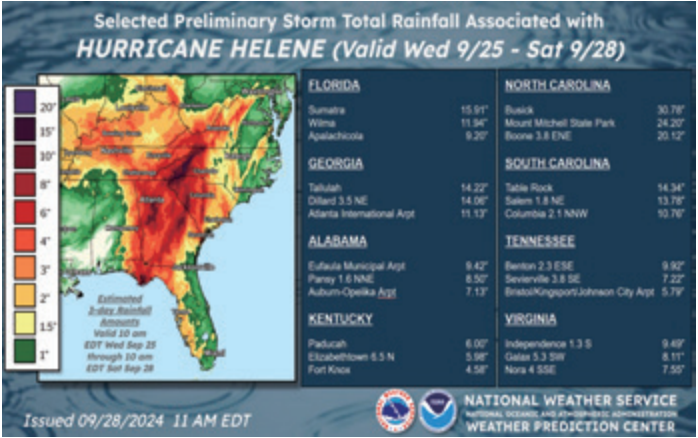
颶風海倫於 9 月 25 日至 28 日的總累積雨量圖（資料來源：NWSWPC）
