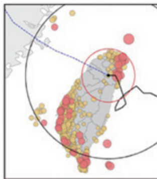
B 7月25日02:00陣風監測
