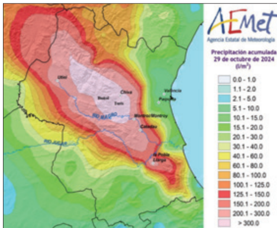
瓦倫西亞省 10 月 29 日累積降雨量情況 (資料來源：AEMET)
