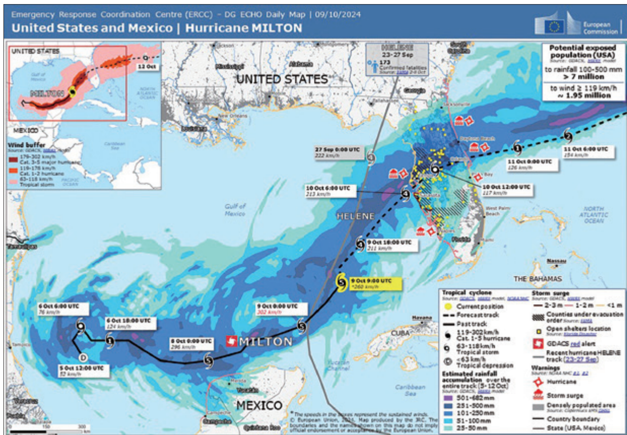
颶風米爾頓 (Milton) 路徑圖 (資料來源: ERCC)
