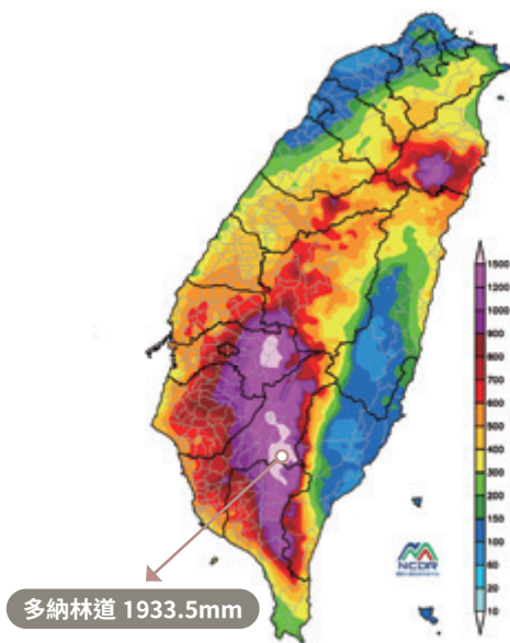
凱米颱風警報期間累積雨量分布圖
