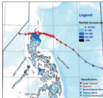
E 萬宜颱風
