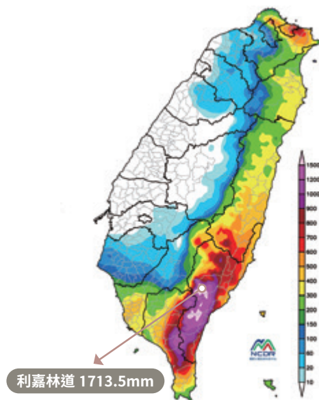
山陀兒颱風警報期間累積雨量分布圖
