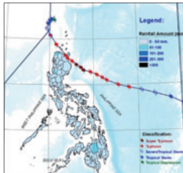
F 天兔颱風
