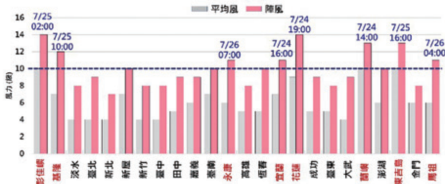
A 測站最大平均風與陣風
