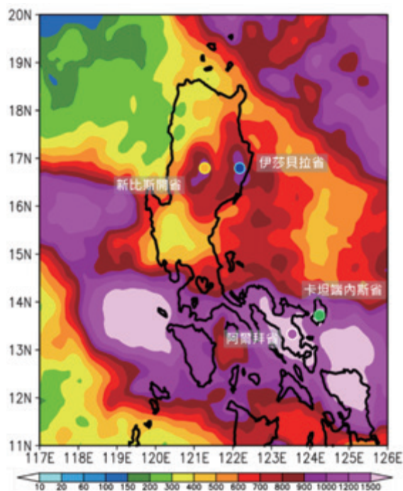
2024 年 10 月 20 日至 11 月 20 日之 GPM 衛星雨量估計 (資料來源：美國國家航空暨太空總署，繪製：災防科技中心)
