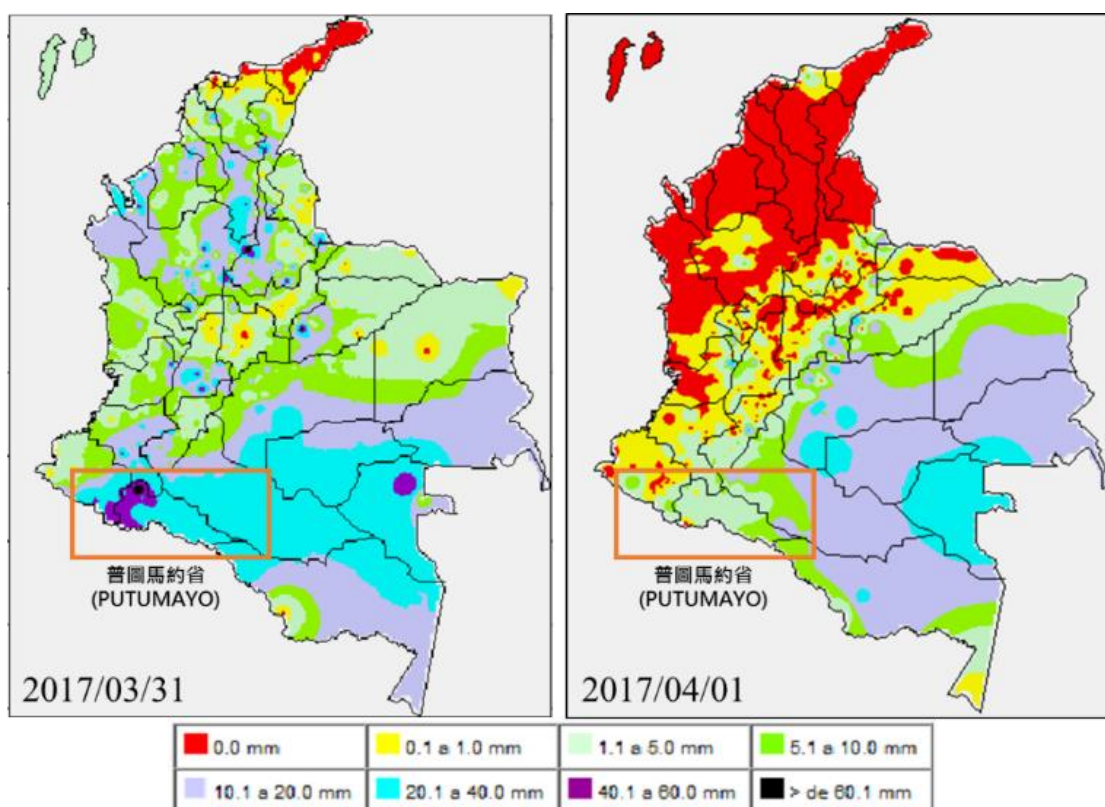
圖 2 哥倫比亞日累積雨量分佈，左圖為 3 月 31 日、右圖為 4 月 1 日（資料來源：IDEAM）
