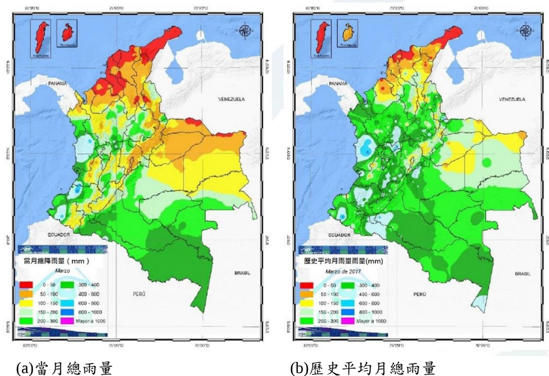
圖 1 哥倫比亞降雨分佈（資料來源：IDEAM）
